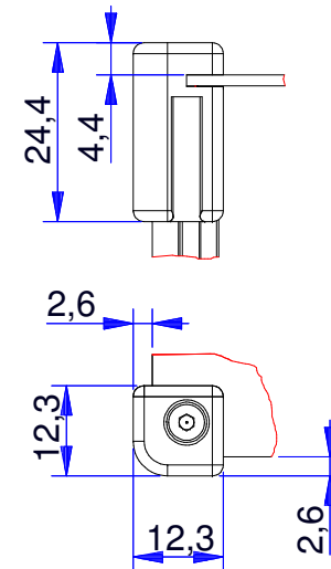
Detail Eckstück
