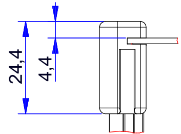
Detail Eckstück
