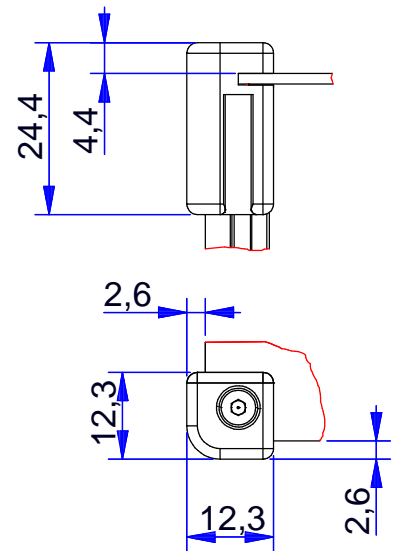
Detail Eckstück
