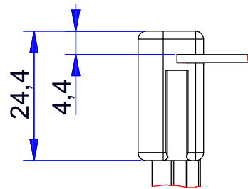
Detail Eckstück
