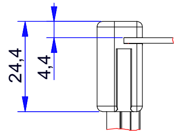
Detail Eckstück
