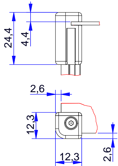
Detail Eckstück
